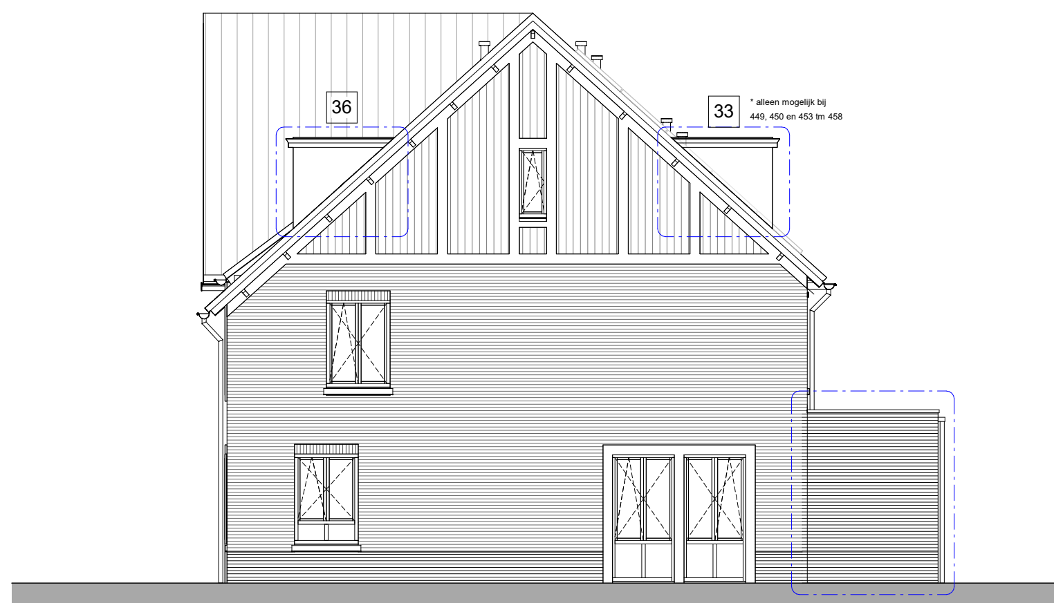
Rechter zijgevel 1 : 100
