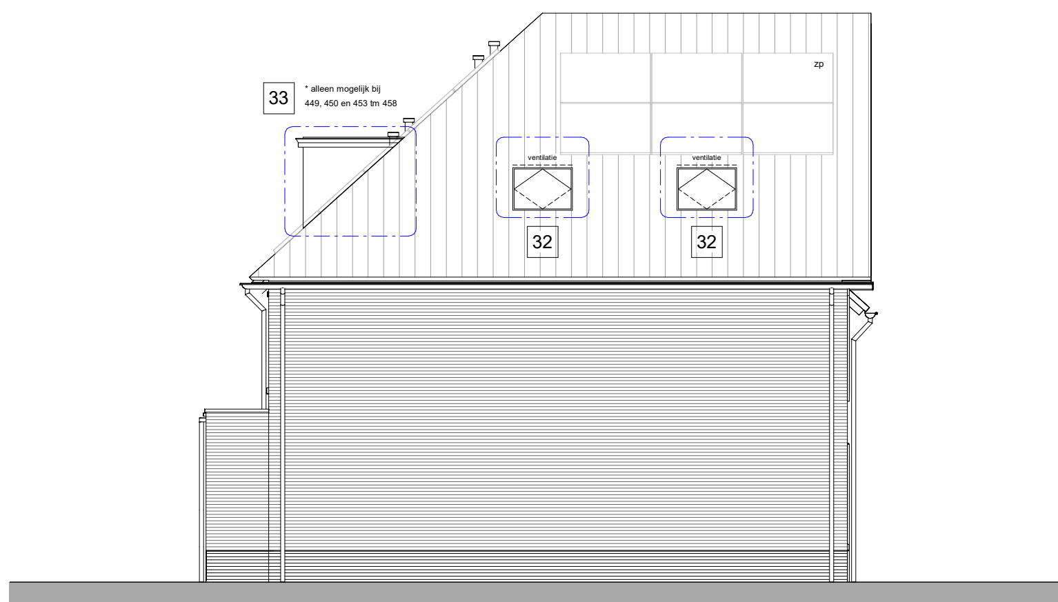
Linker zijgevel 1 : 100
