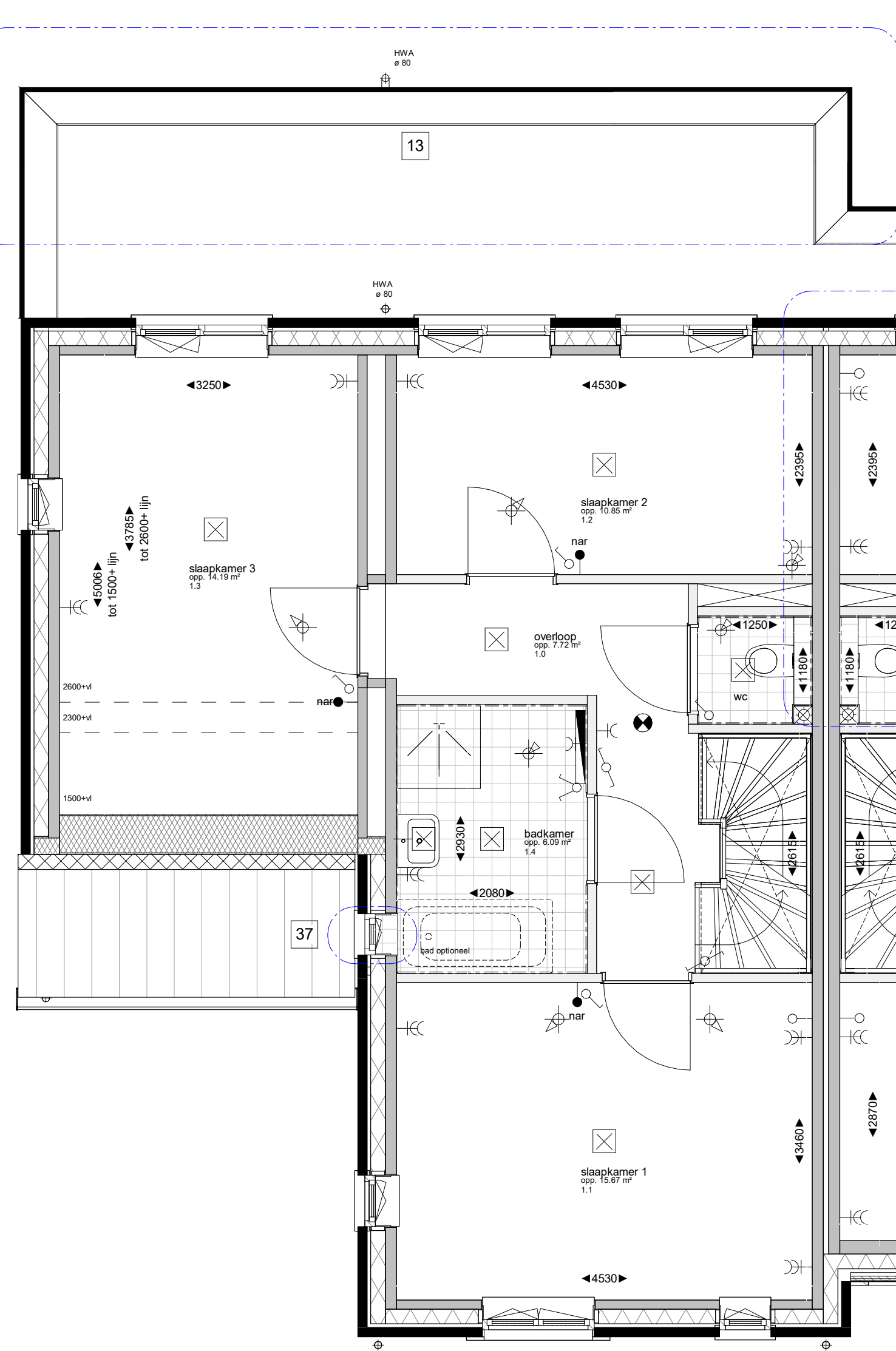
1e Verdieping +2920
