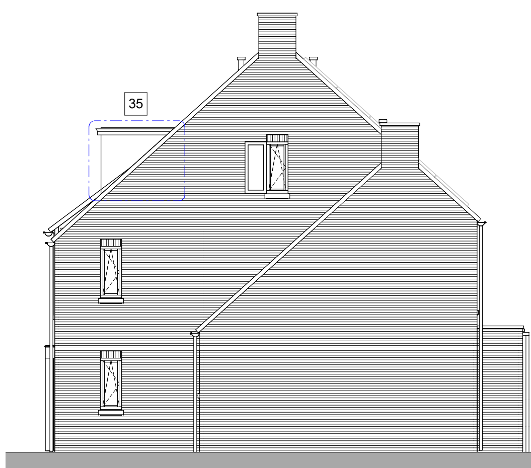
Rechter zijgevel 1:100
