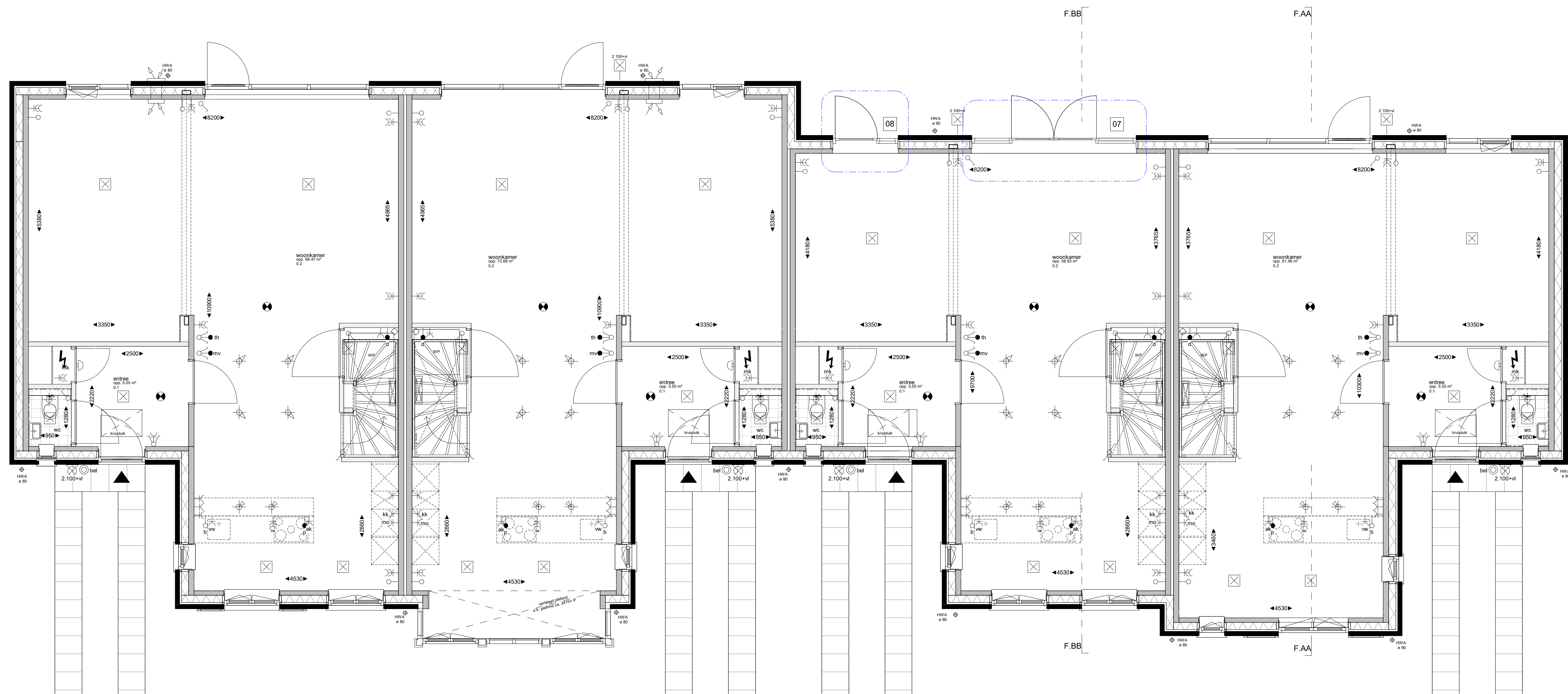
Begane grond Peil=0 1:100
