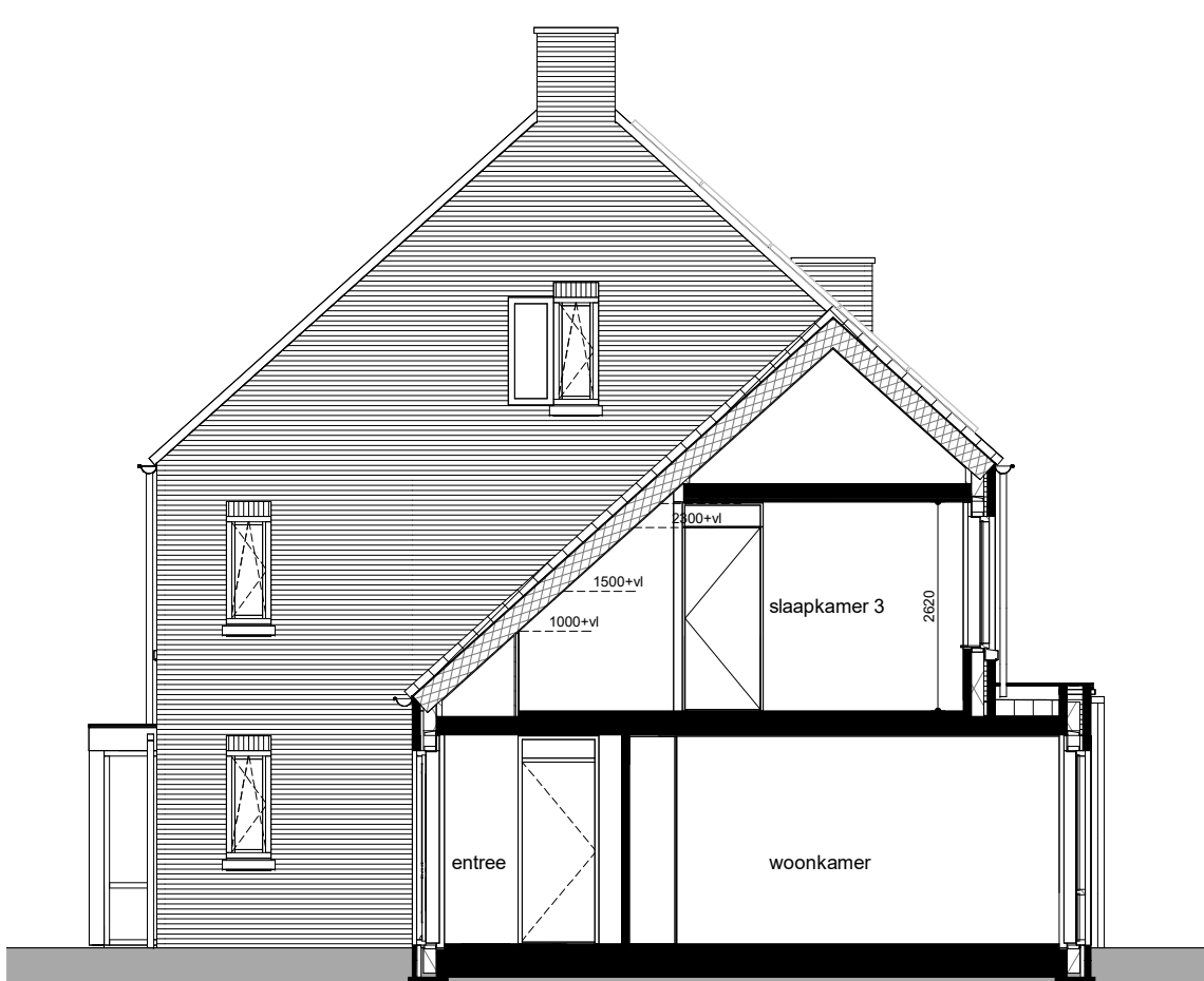
Rechter zijgevel 1:100
