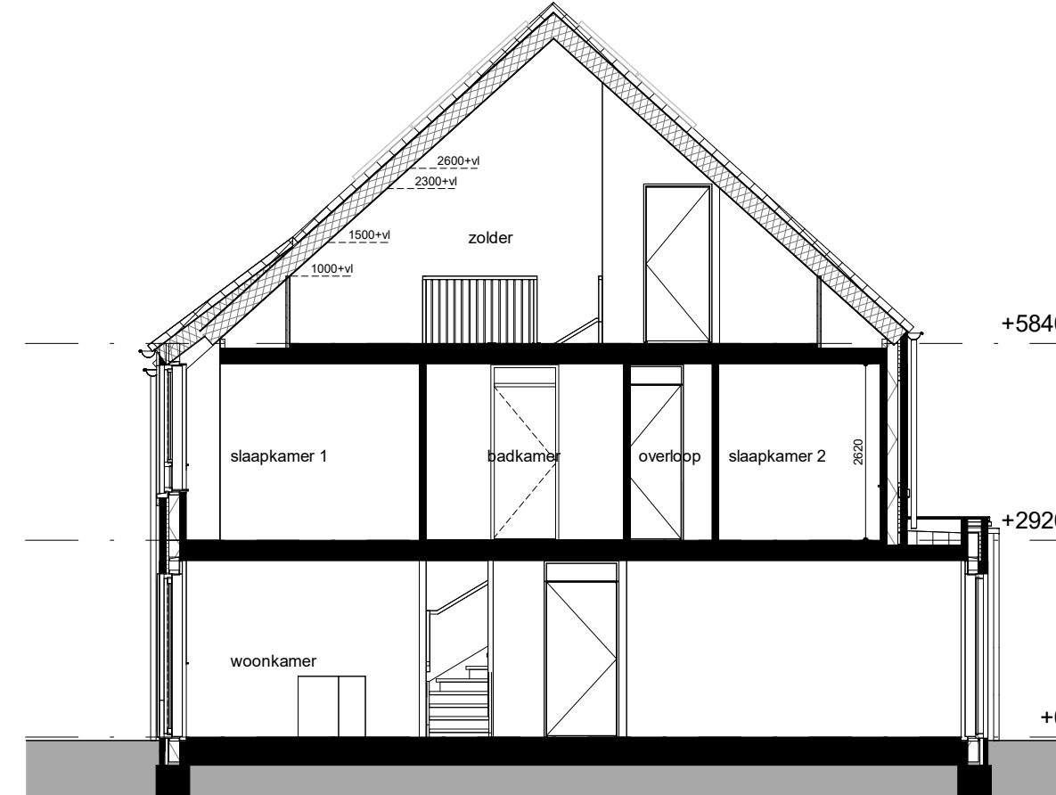
Doorsnede J.BB-J.BB
