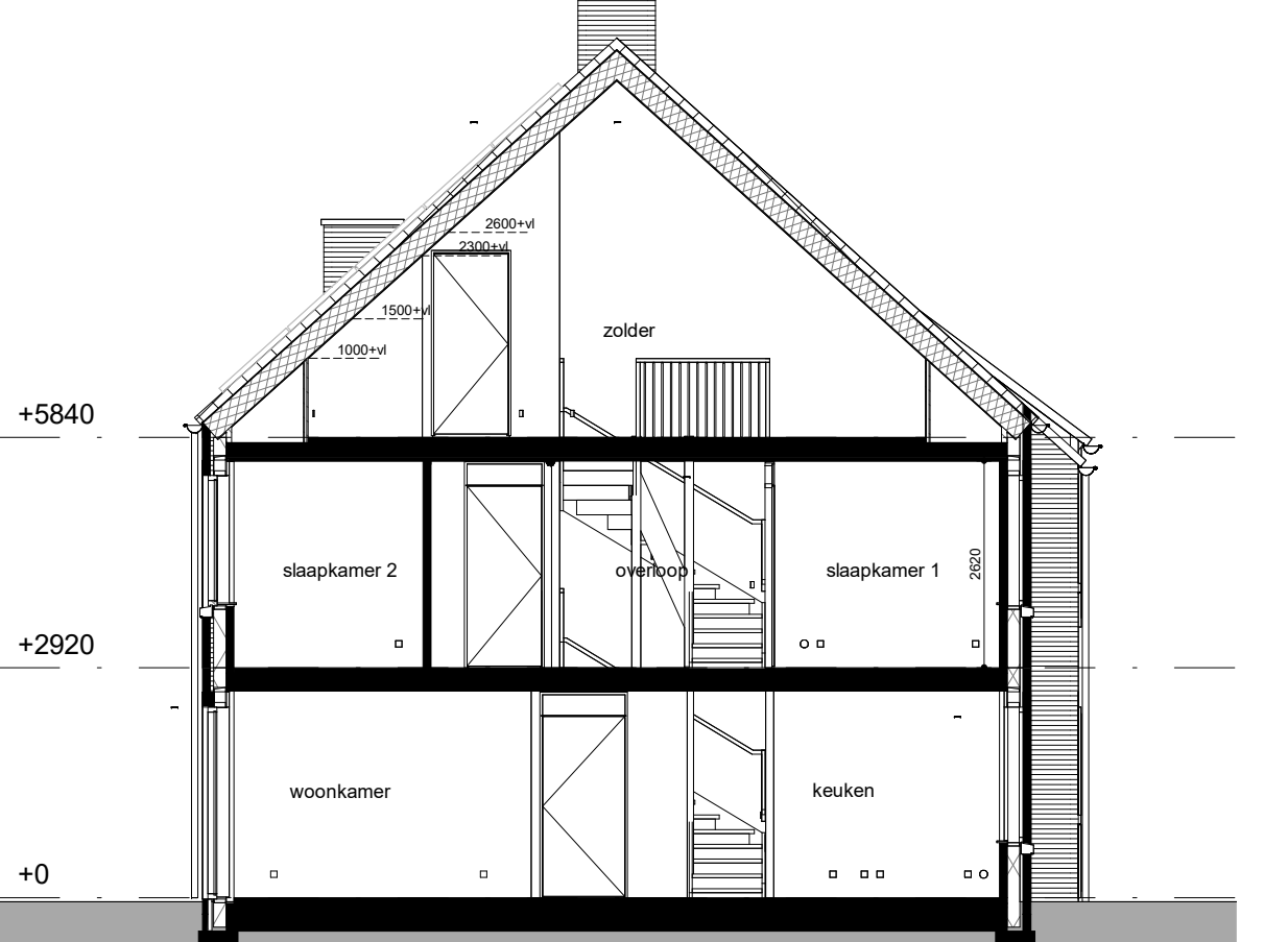
Doorsnede F.BB-F.BB 1:100
