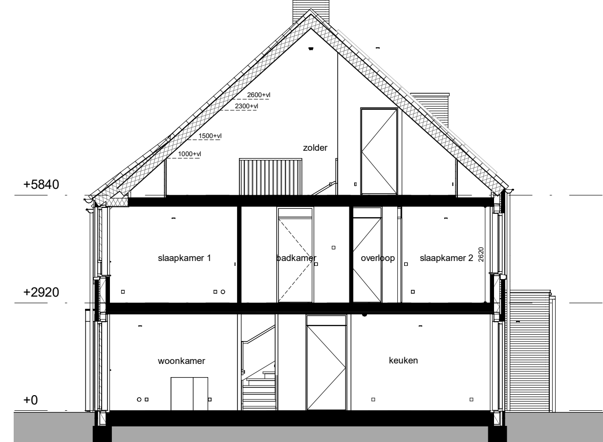
Doorsnede F.AA-F.AA 1:100
