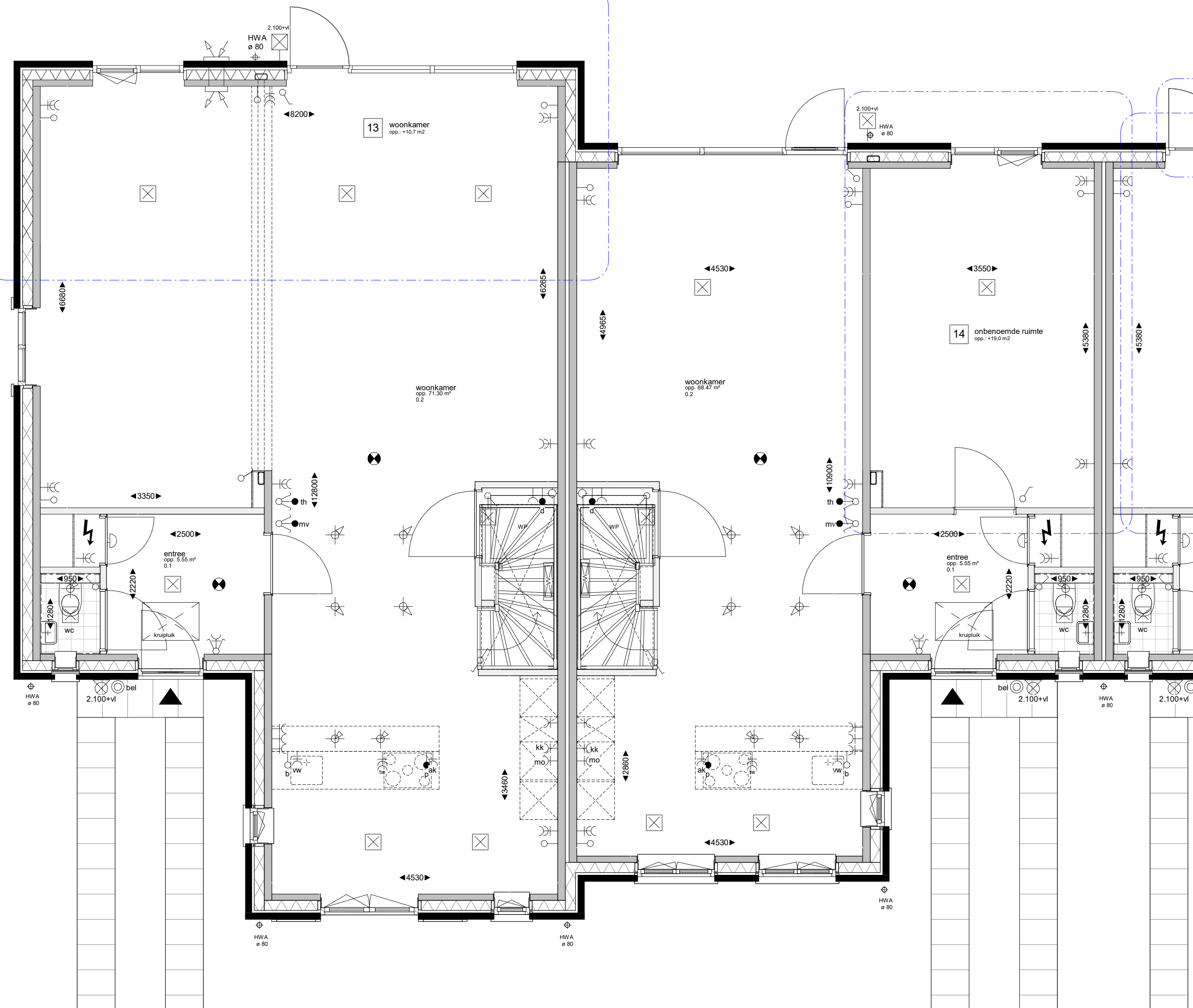
Begane grond Peil=0
