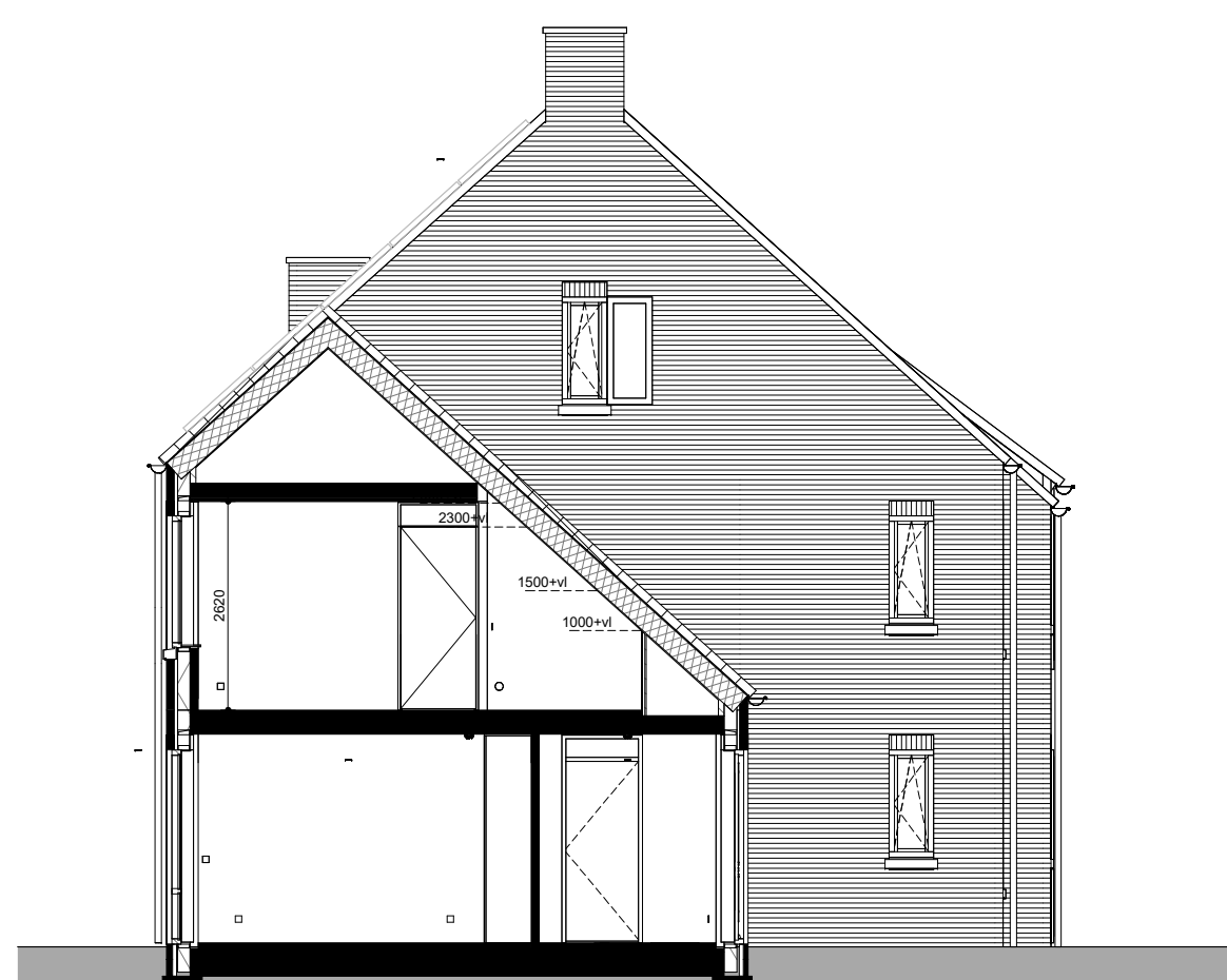
Linker zijgevel 1:100
