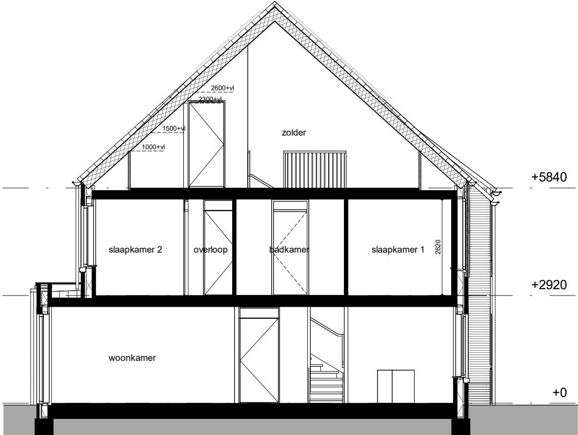
Doorsnede J.AA-J.AA
