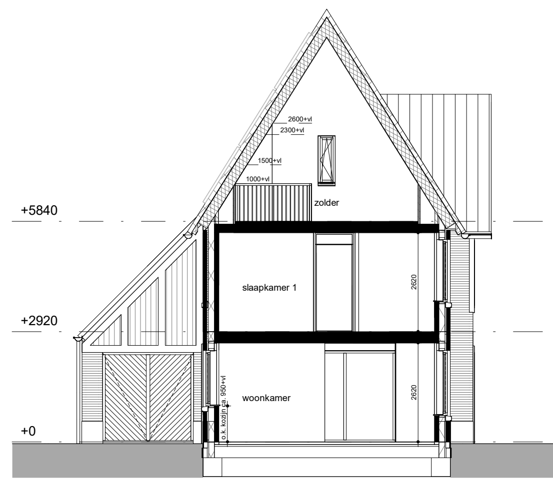
Doorsnede D1.AA-D1.AA 1 : 100
