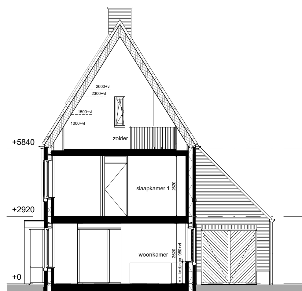
Doorsnede D3.AA-D3.AA 1:100
