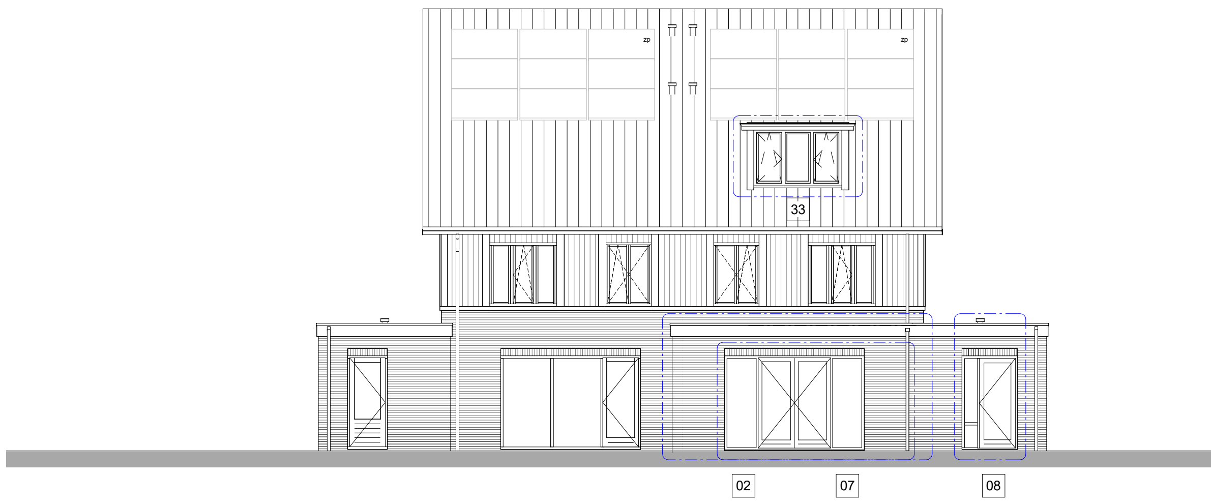
Achtergevel 1:100
