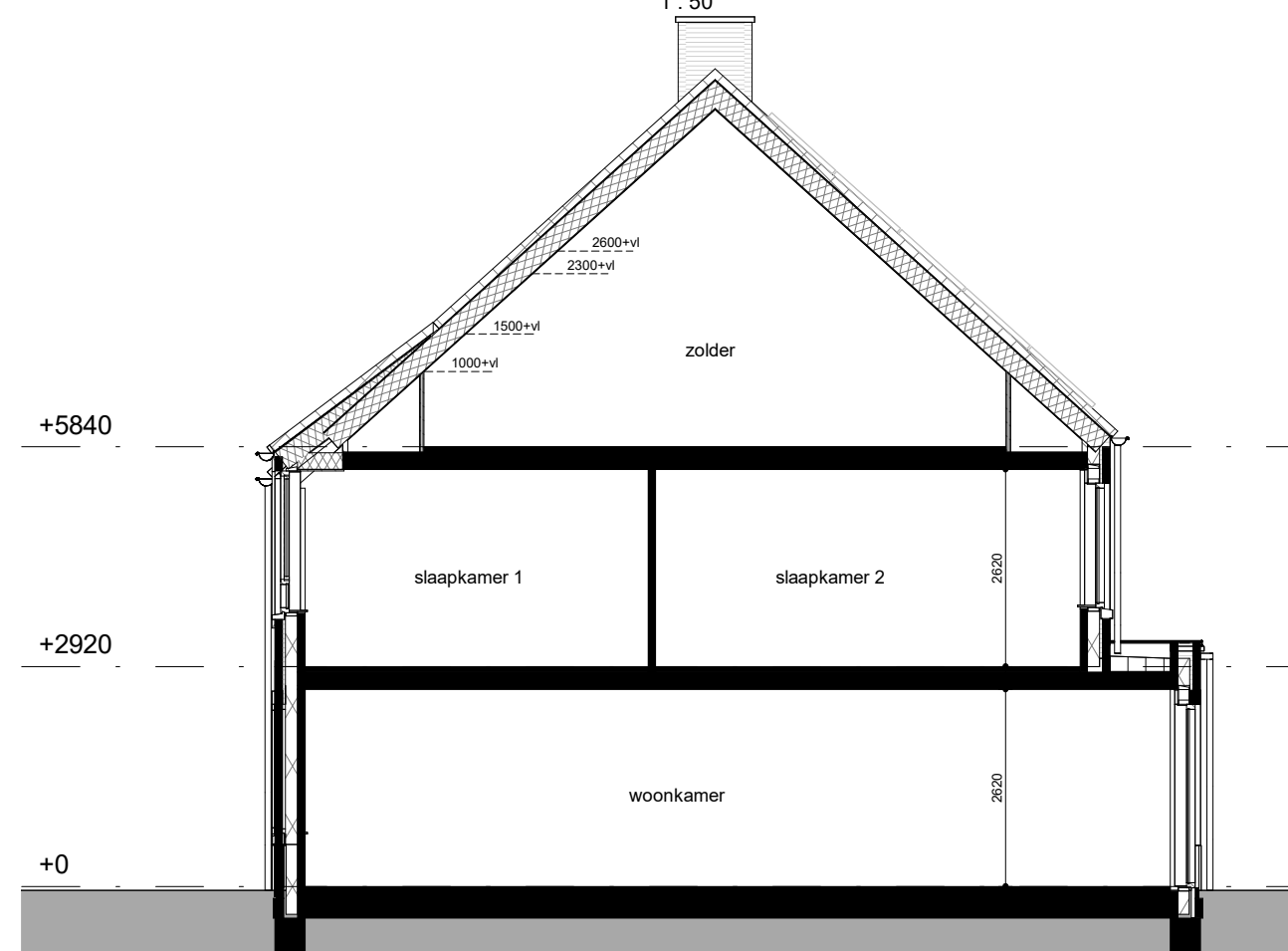
1e Verdieping +2920
