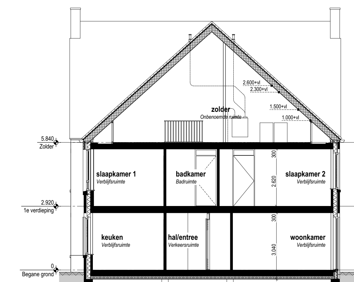
Doorsnede A-A (1:100)
