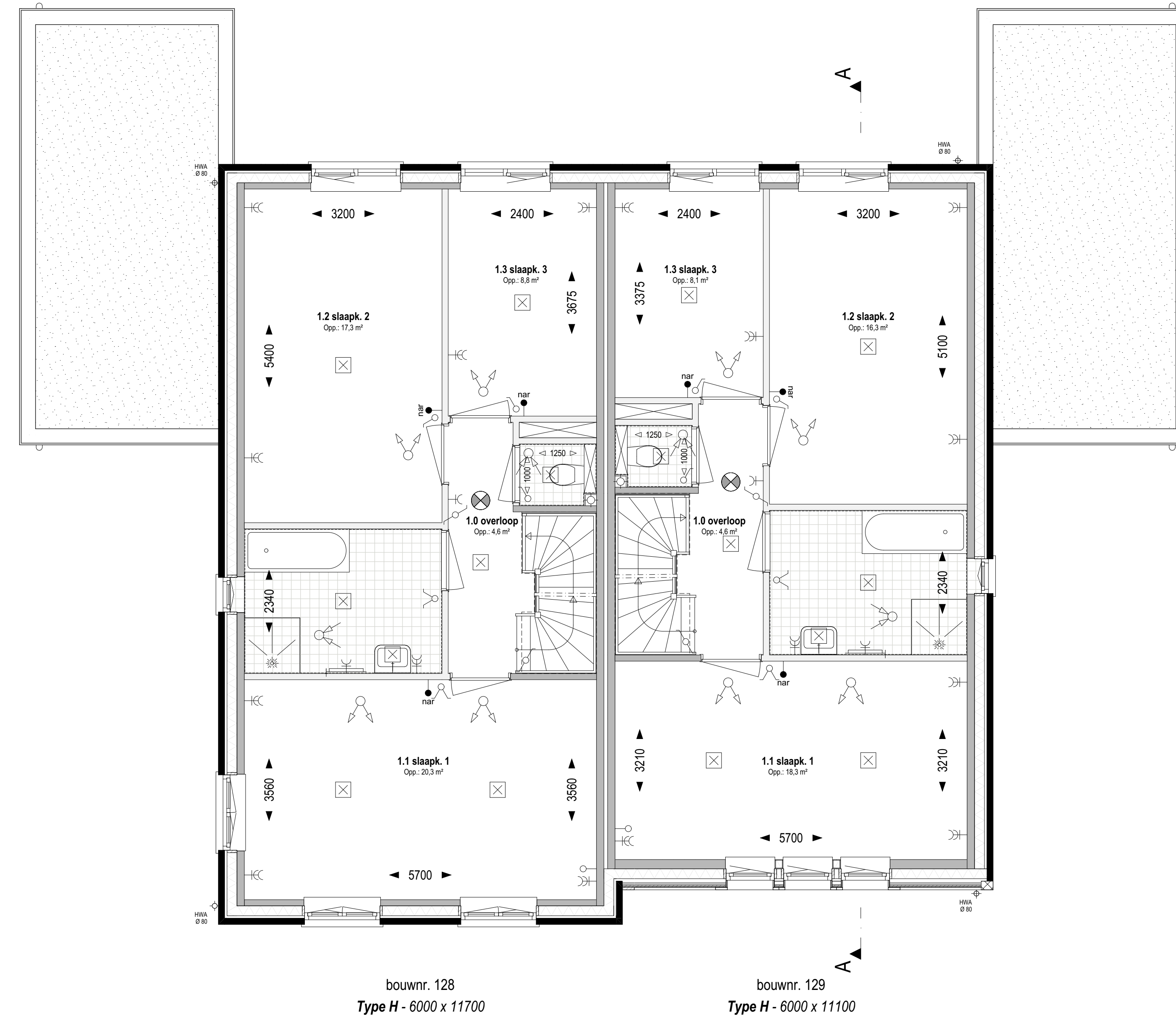
1e Verdieping +2920 (1:50)
