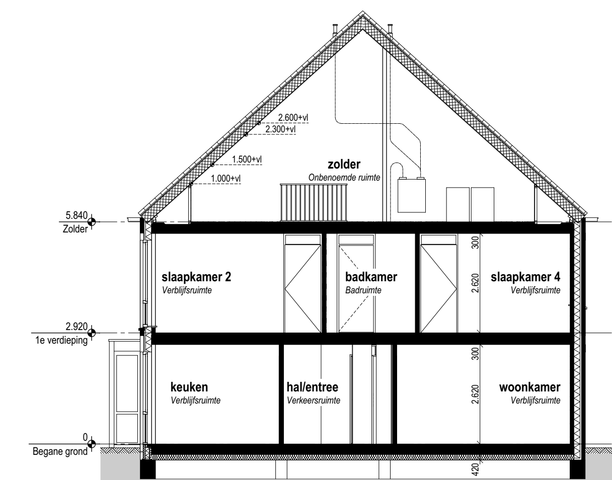
Doorsnede A-A (1:100)
