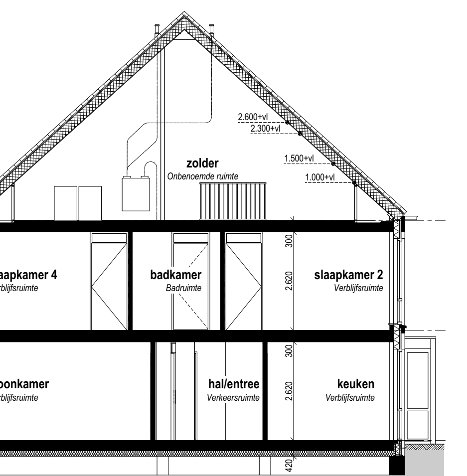
Doorsnede A-A (1:100)
