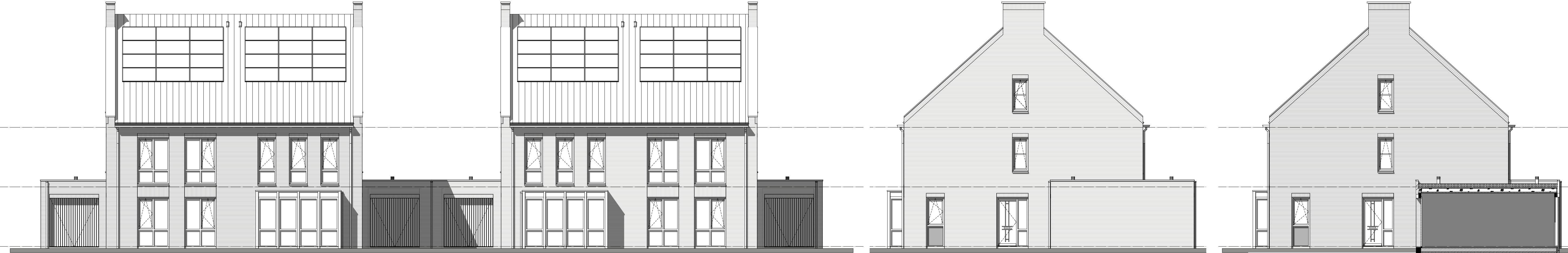
Voorgevel (1:100) Rechter zijgevel (1:100) Linker zijgevel (1:100) Achtergevel (1:100)
